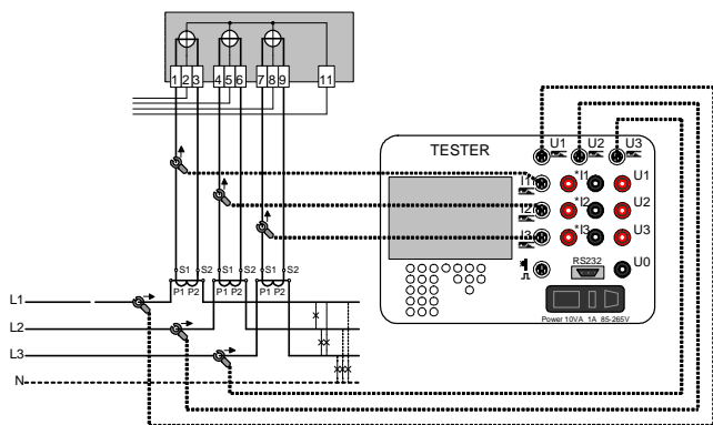
Rys. 4. Układ do pomiaru błędów przekładnika Fig. 4. Circuit for error measurement of current transformer
