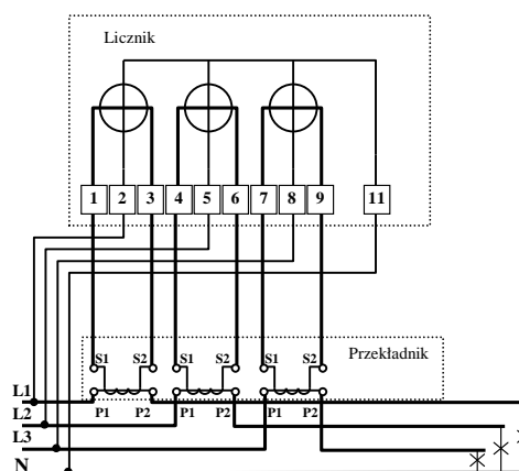
Rys. 1. Układ półpośredni pomiaru energii
