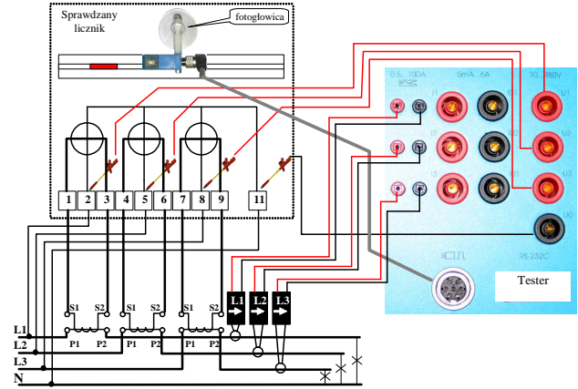
Rys. 2. Układ do pomiaru błędów układu półpośredniego
