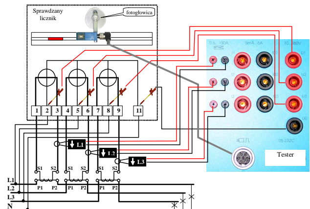
Rys. 3. Układ do pomiaru błędów licznika
