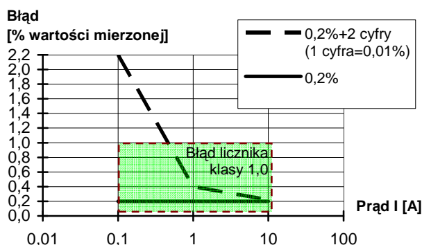
Rys. 1. Wykres błędów testera dla dwóch rodzajów specyfikacji dokładności
