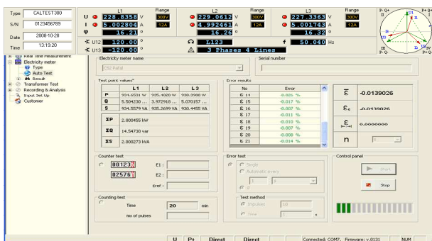
Rys. 6. Ekran automatycznego testu błęd licznika
